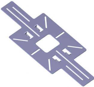
Quermontage des Universalblechs
